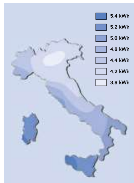
Radiazione solare media annua su un piano inclinato di 30° rivolto a sud [kWh/m²].
