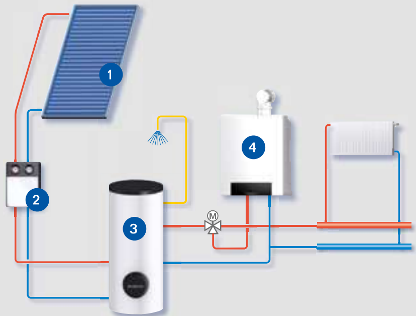
Impianto solare a circolazione forzata
